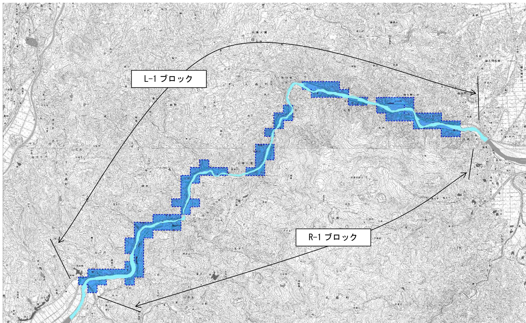
様式-1 氾濫ブロック分割図 水系名：阿武隈川水系 河川名：阿武隈川
