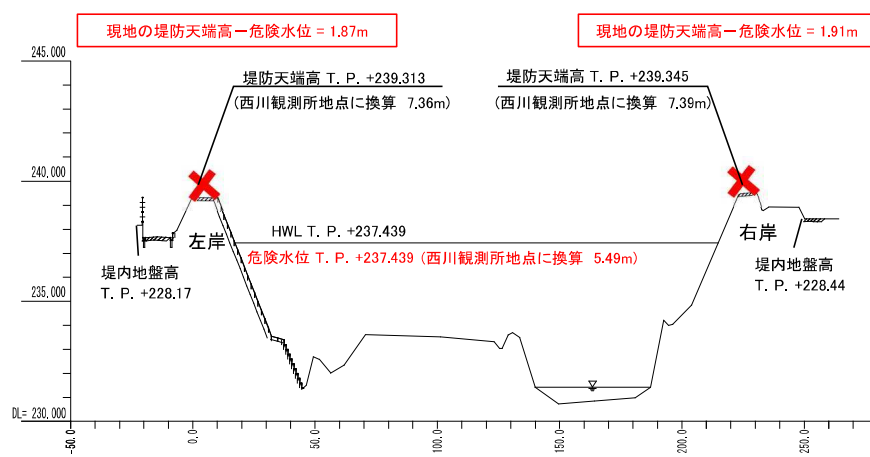
○危険箇所付近の横断面図(1.0k付近)
