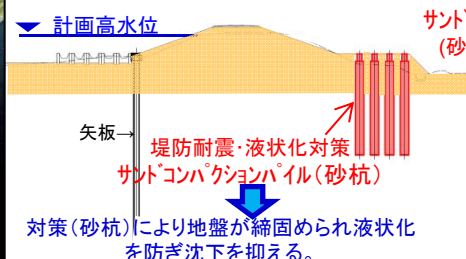
▲対策工断面図
