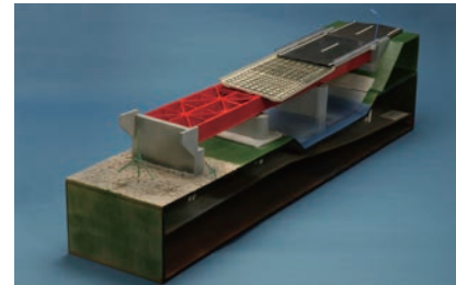
アイデア賞 | 3径間連続複合橋 構造模型
