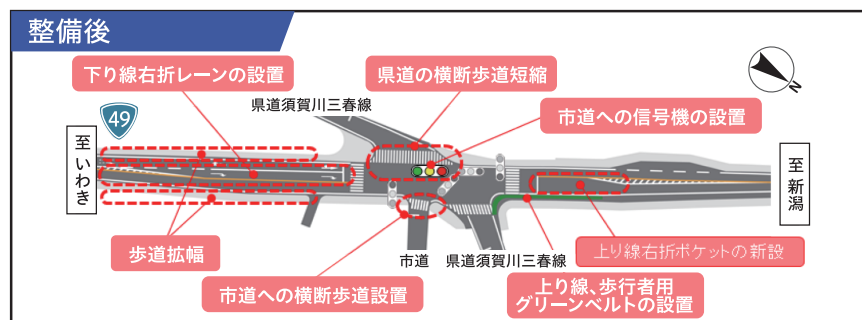
（下り線）県道への右折レーン設置
