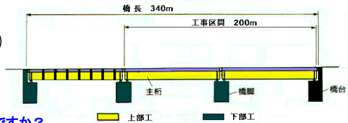
泉高架橋略図 340m
