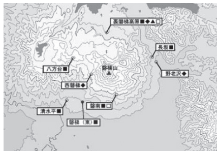
▲磐梯山の火山観測点配置
