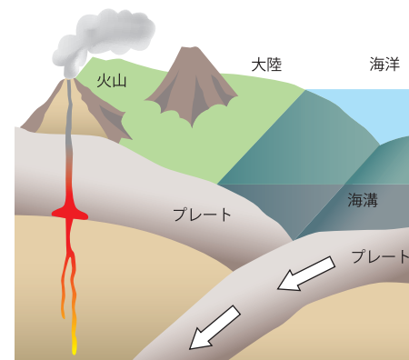
▲プレートと火山の関係図
