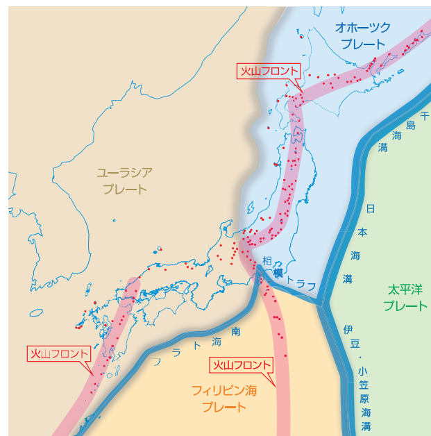
▲日本周辺のプレートと火山帯
