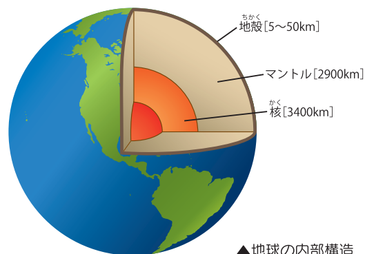
▲地球の内部構造
