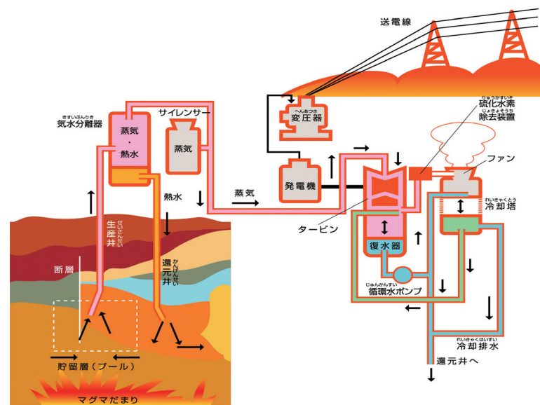
▲地熱発電図
