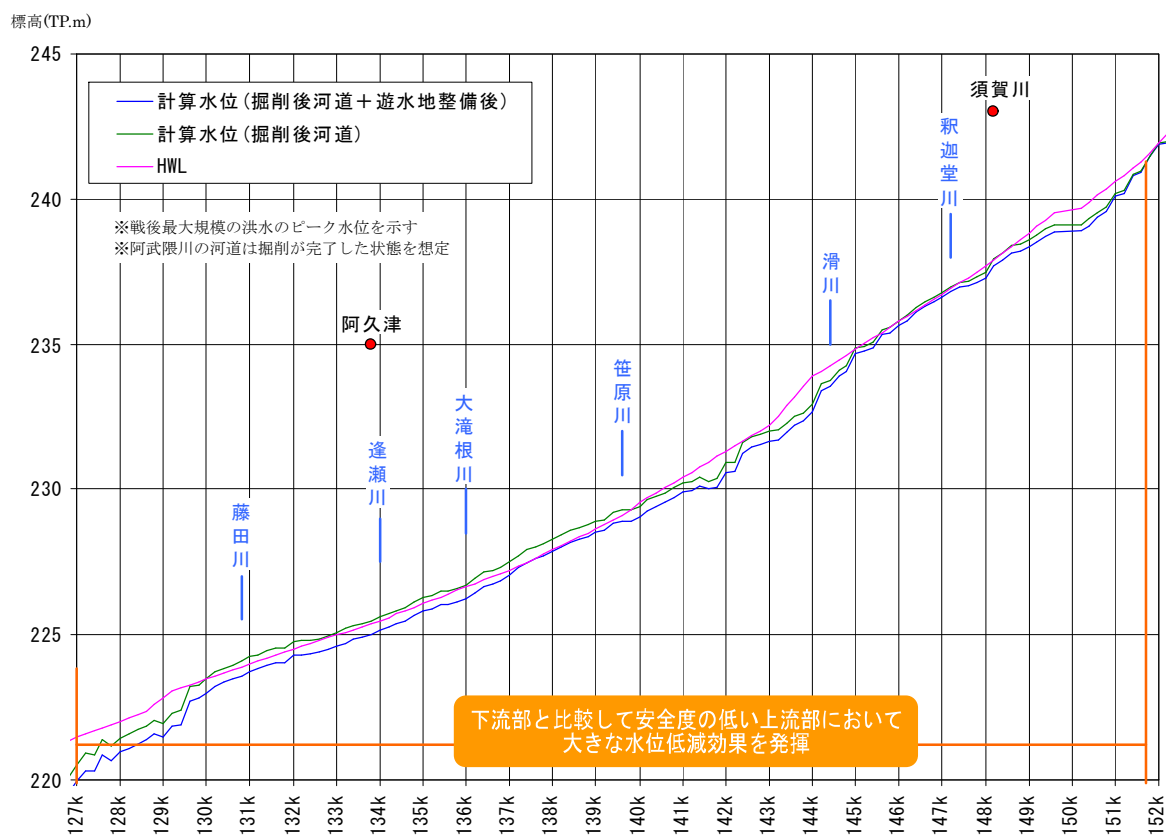
図 5-12 遊水地整備等による水位低減効果
