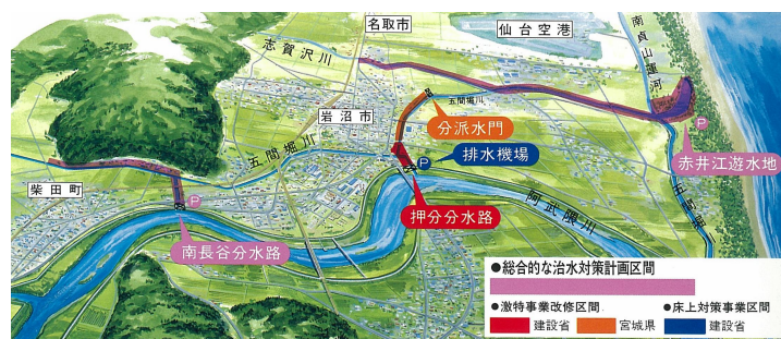
五間堀川の総合的な治水計画 ～宮城県と国土交通省の分担～
