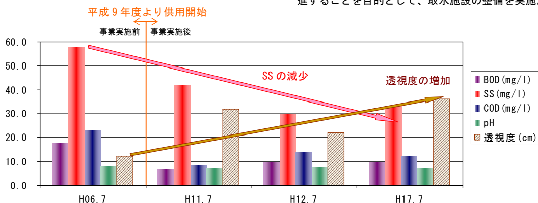
図3-26 徳定川浄化事業実施後の古川池水質改善効果 (事業実施H9)
