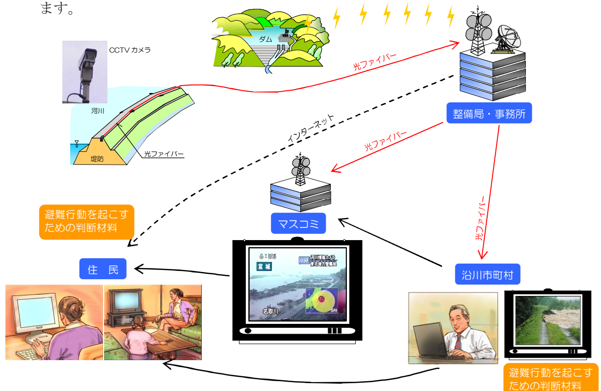
図5-34 ITを活用した河川情報の提供イメージ
