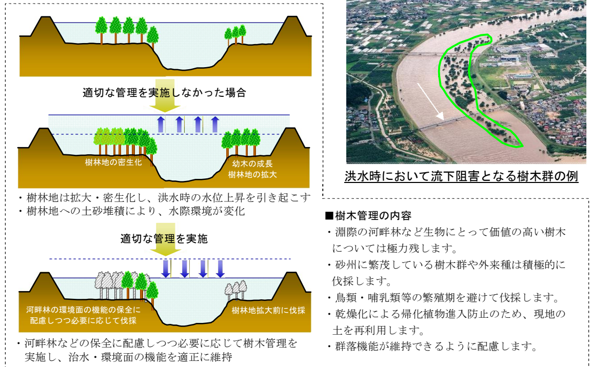
図 5-28 樹木管理イメージ（断面図）
