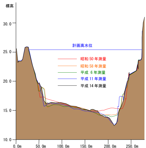
図 5－26 横断形状経年変化 【河口より 38.0km 付近】
