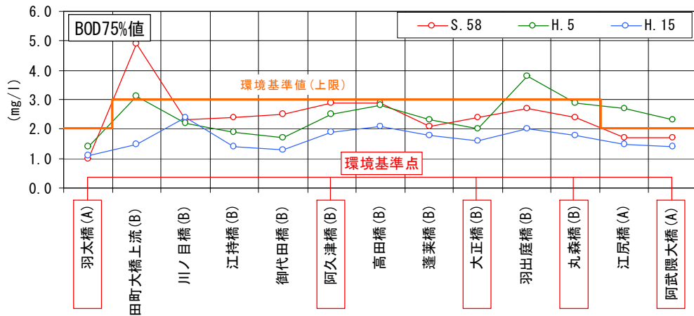
図3-20 阿武隈川におけるBOD75%値の経年変化
