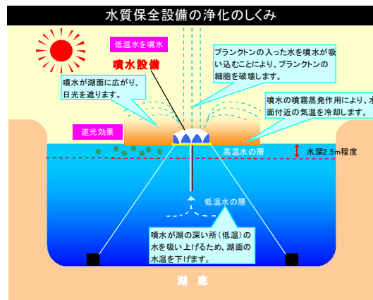
水質保全設備の浄化のしくみ
