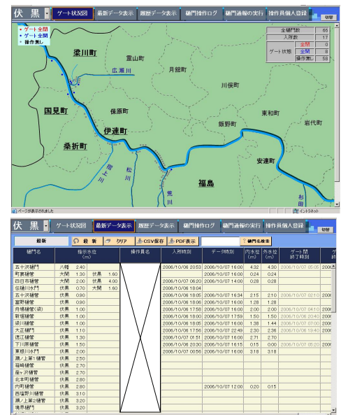
図5-30 樋門情報管理システム
