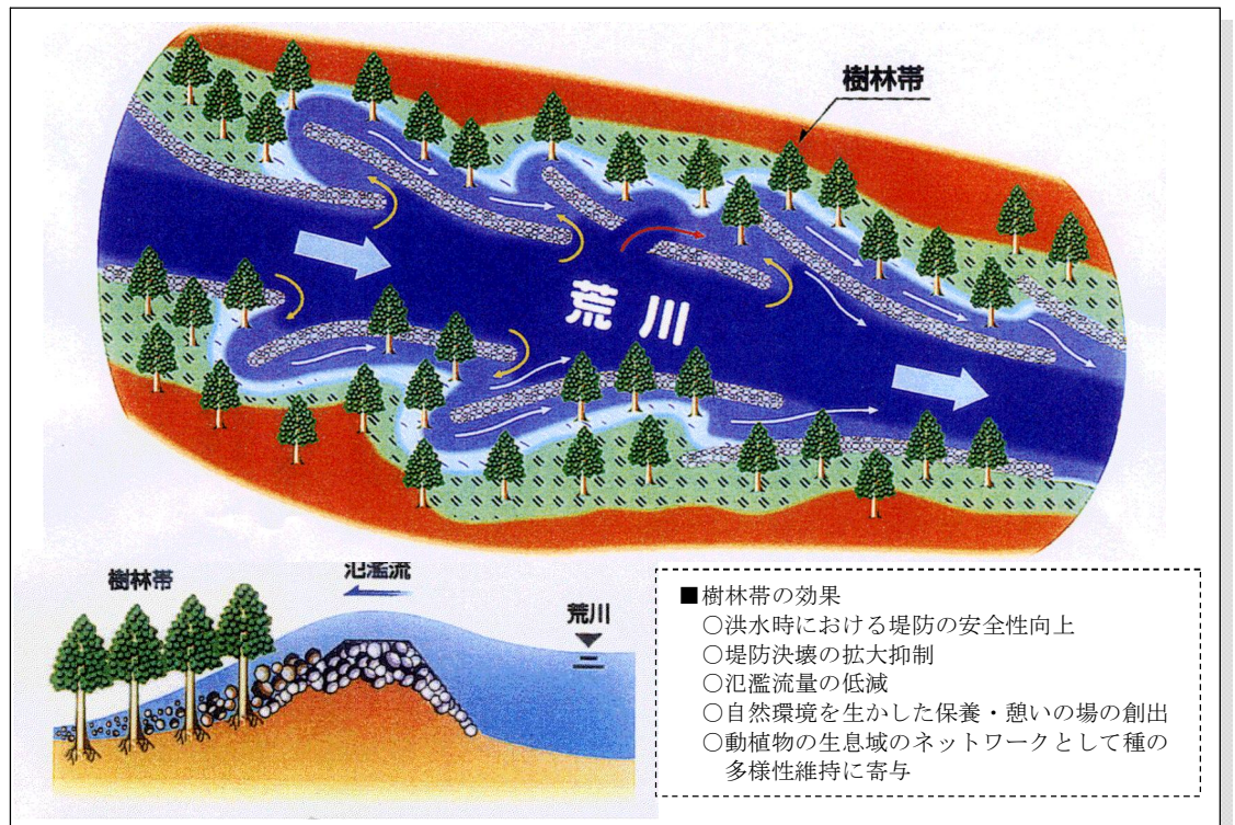
図5-27 樹林帯の概要（支川荒川）
