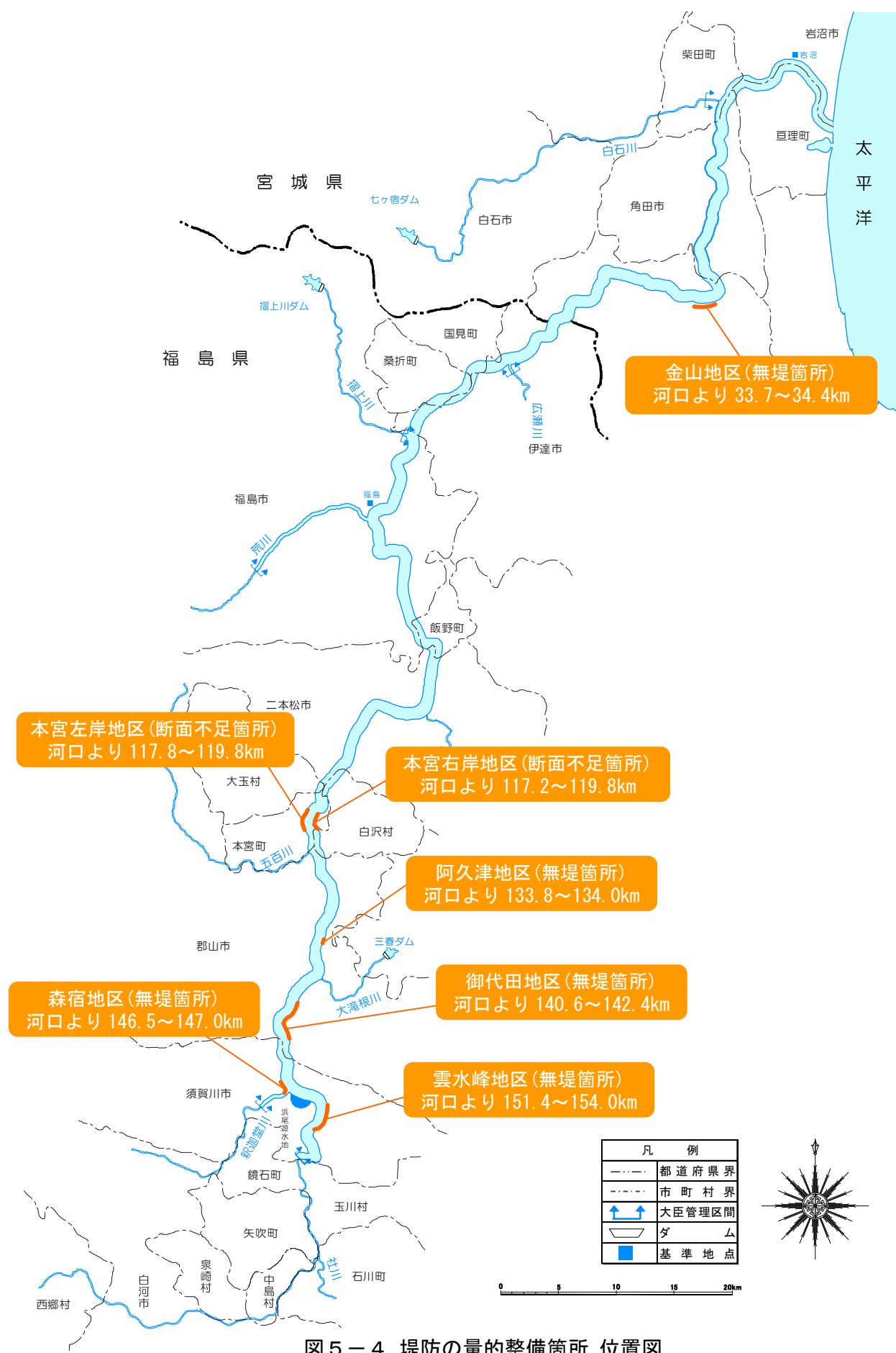
図5－4 堤防の量的整備箇所 位置図
