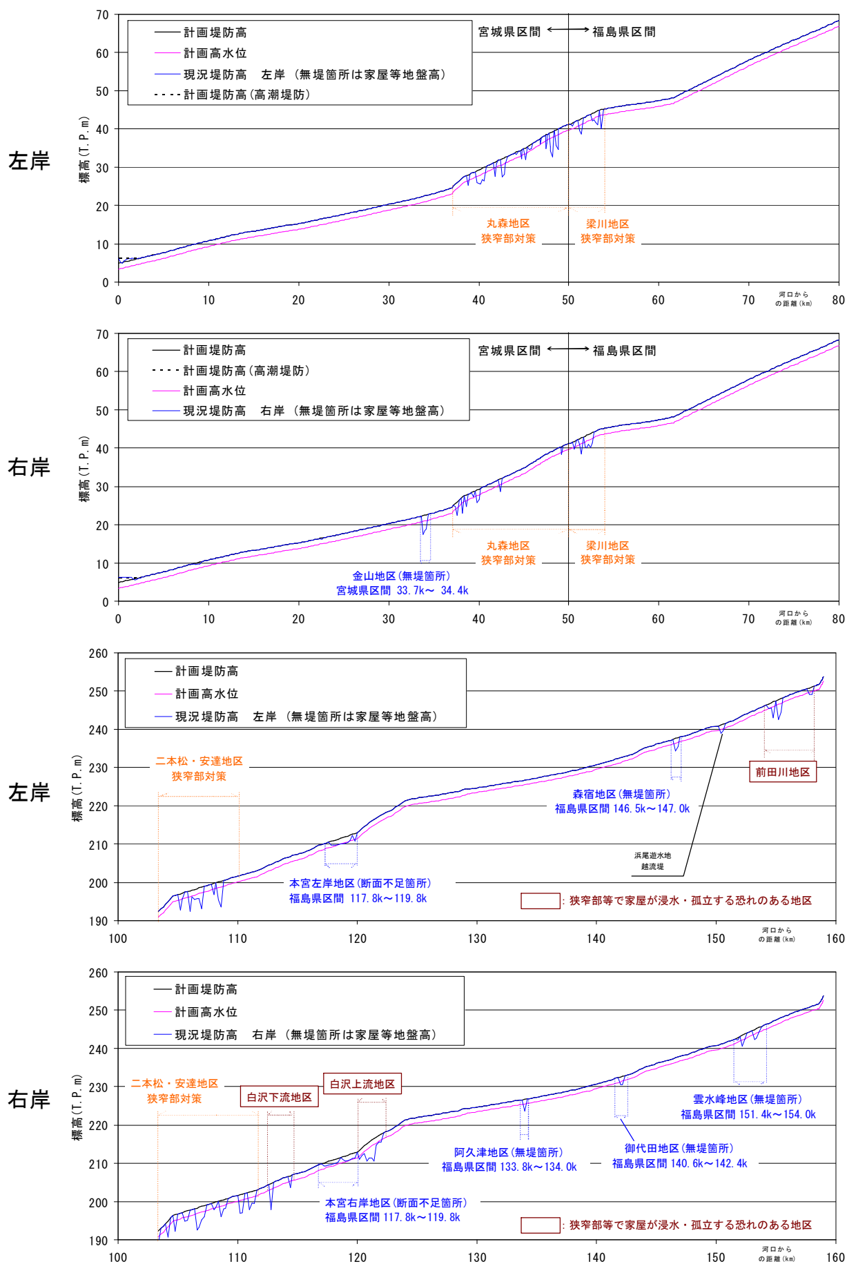
図5-3 現況堤防高
