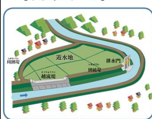
【平常時のイメージ】
