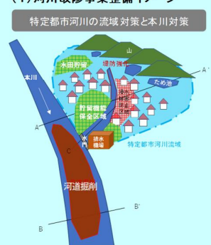
(1) 河川改修事業整備イメージ
