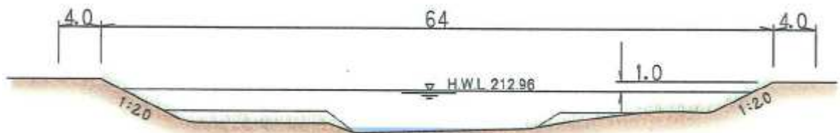
図13 屋代川代表横断図（吉野川合流点から上流 0.3km、単位：m）
