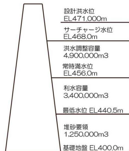
図15 貯水池容量配分図
