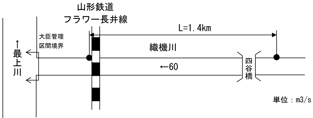
図21 計画流量配分図（織機川）
