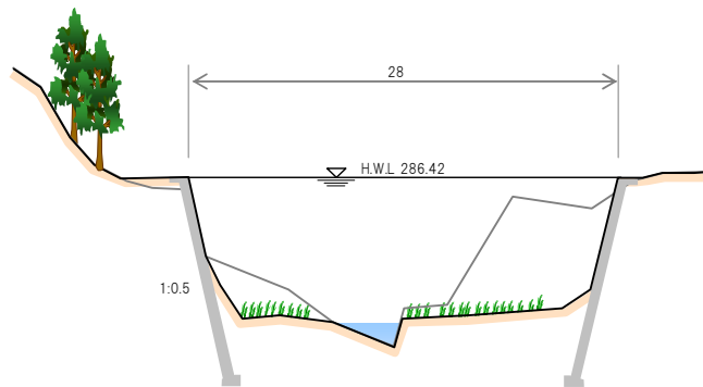
図12 吉野川代表横断図（直轄管理区間から上流 12.3km、単位：m）
