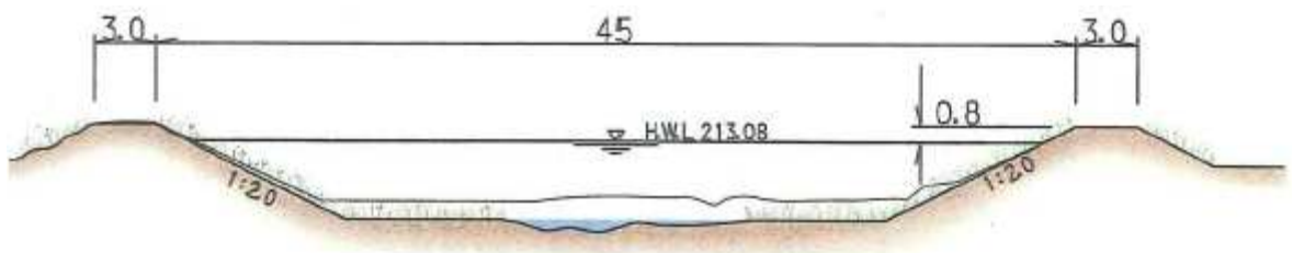
図11 吉野川代表横断図（直轄管理区間から上流 0.6km、単位：m）
