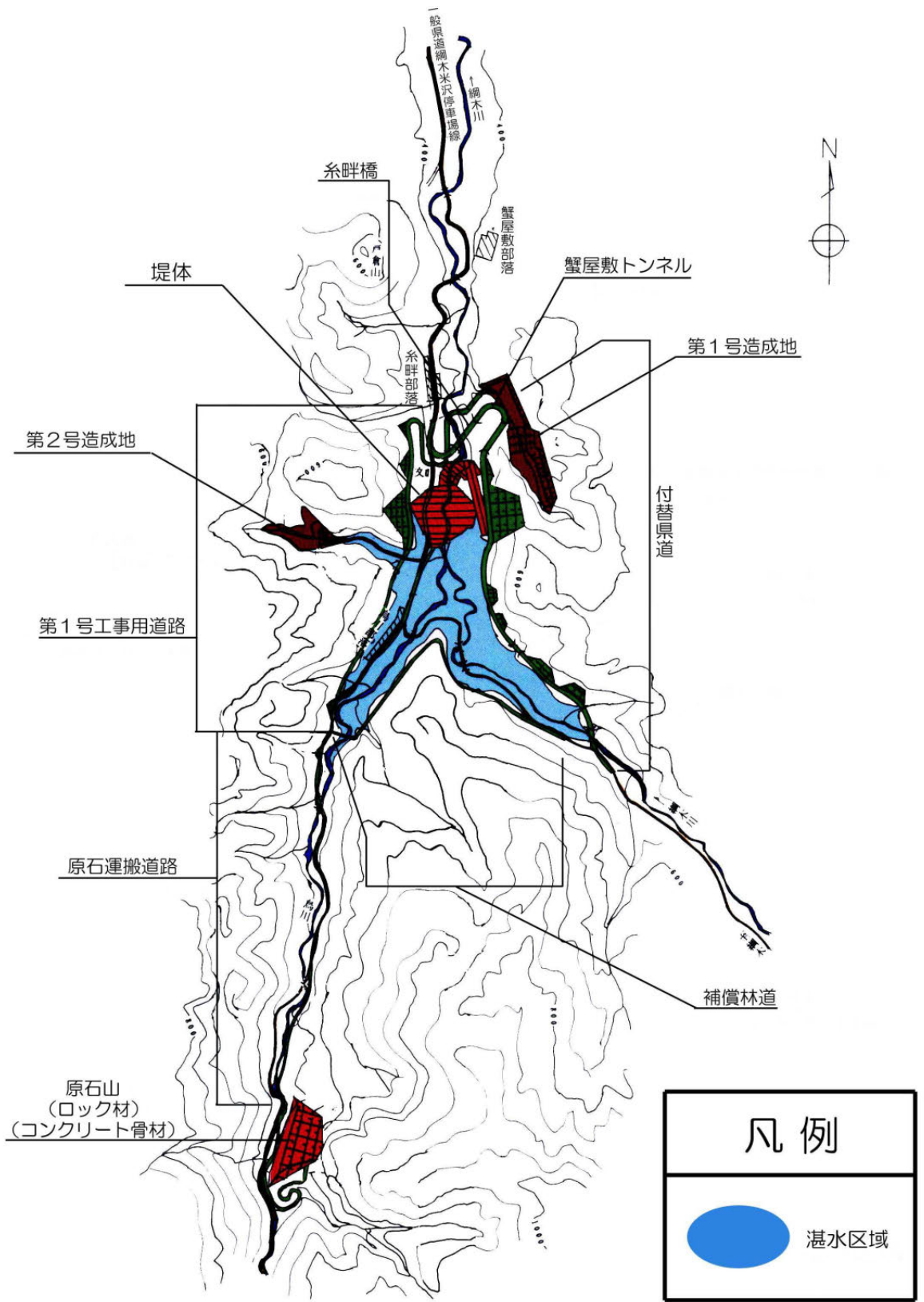
図16 網木川ダム湛水区域図
