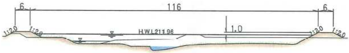
図10 吉野川代表横断図（直轄管理区間から上流 0.1km、単位：m）
