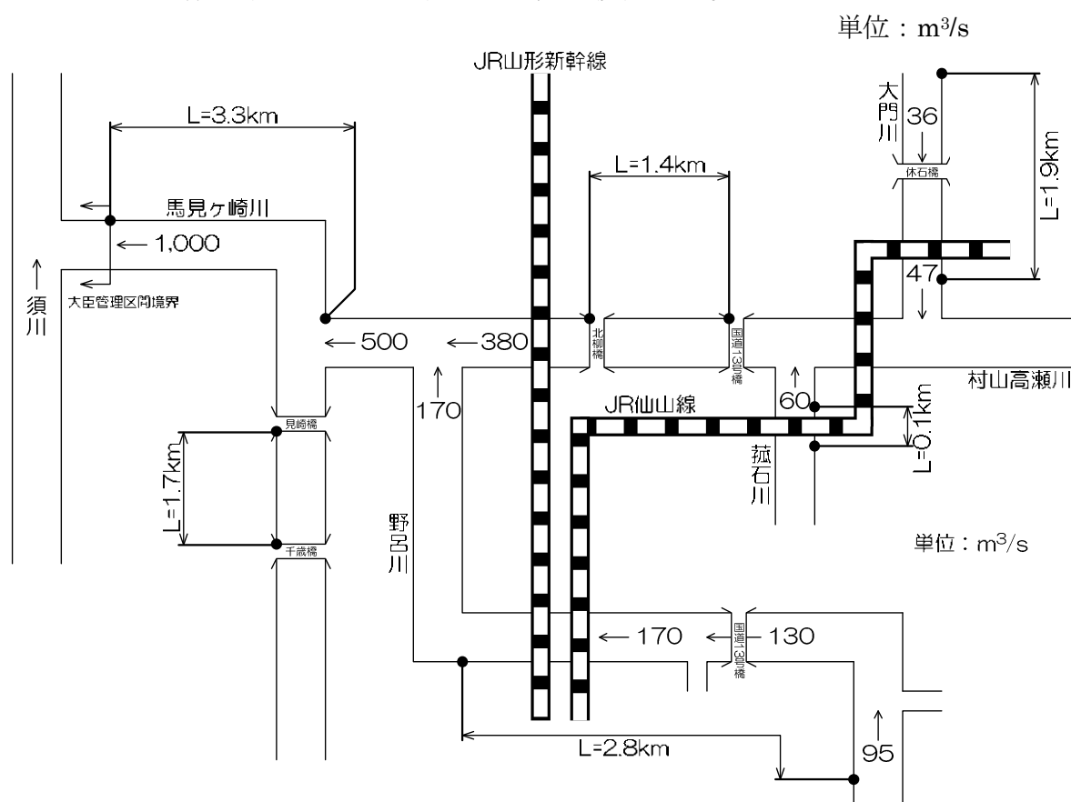
図28 計画流量配分図（馬見ヶ崎川流域）
