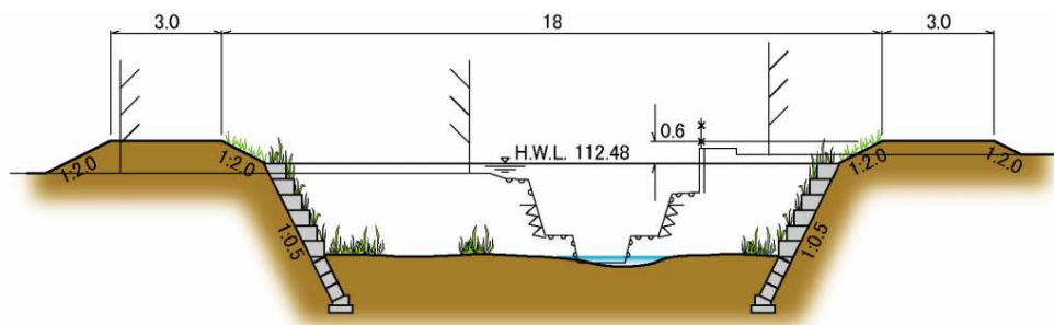
図32 野呂川上流代表断面図 (村山高瀬川合流点から上流 2.6km、単位：m )
