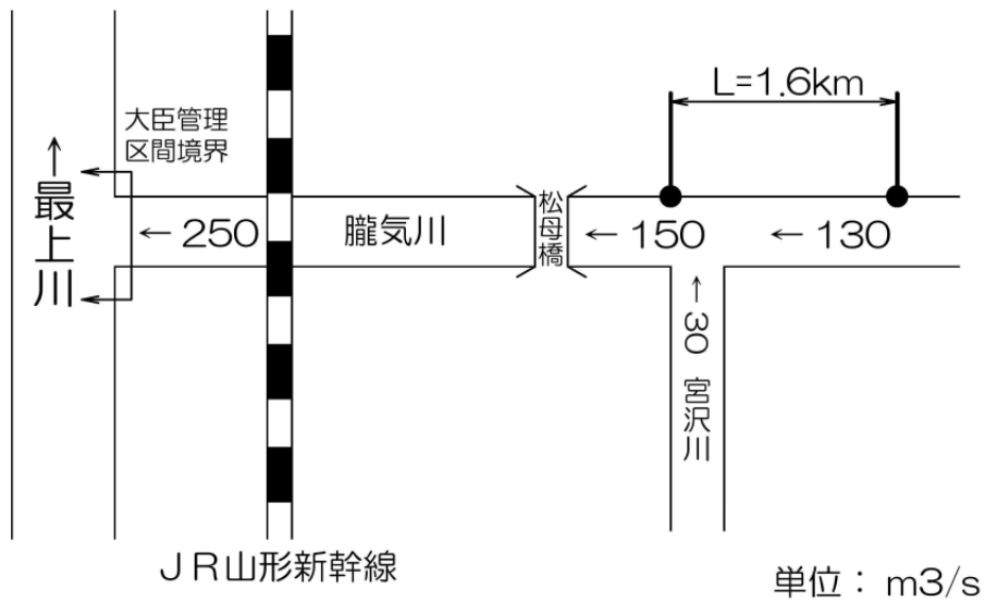
図2 計画流量配分図（朧気川）
