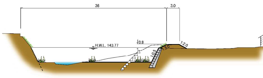
図39 月布川代表断面図（最上川合流点から上流 9.2km、単位：m）
