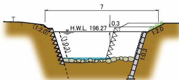
図34 大門川上流代表断面図 (村山高瀬川合流点から上流 2.0km、単位：m )
