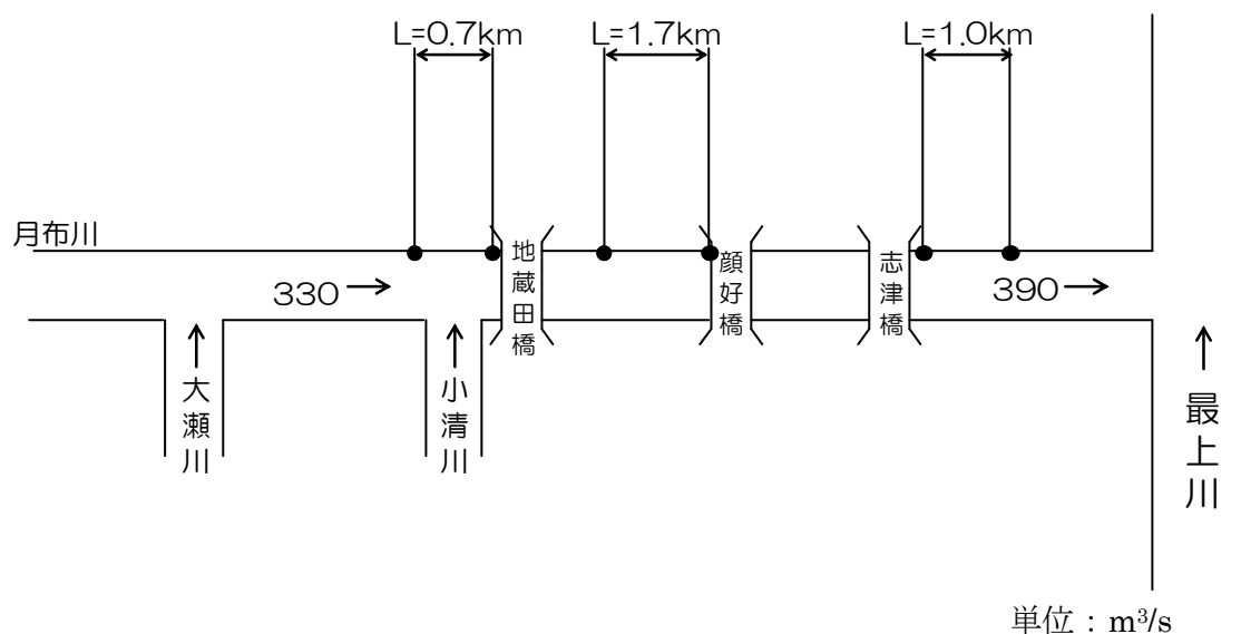
図38 計画流量配分図（月布川）
