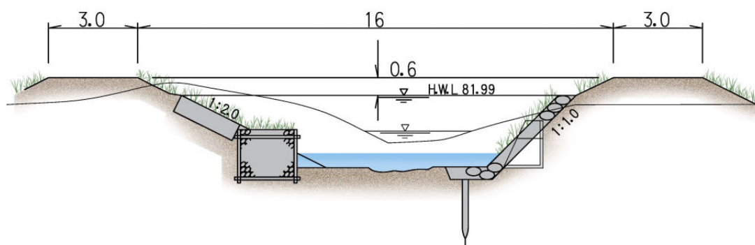
図9 荷口川代表断面図（小見川合流点から上流 0.2km、単位：m）
