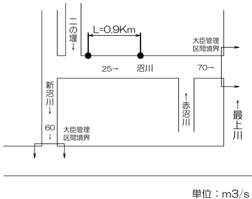
図17 計画流量配分図（沼川）
