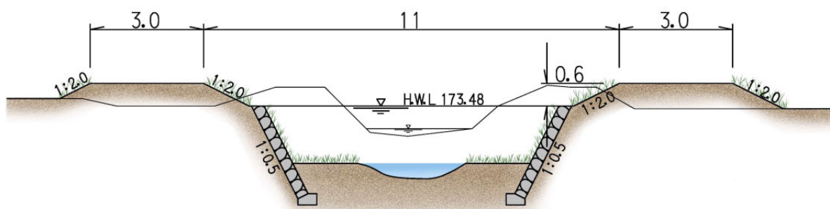
図33 大門川下流代表断面図 (村山高瀬川合流点から上流 0.7km、単位：m )
