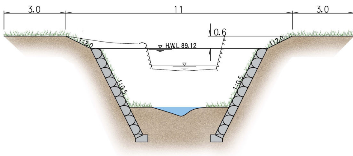
図35 菰石川代表断面図 (村山高瀬川合流点から上流 0.2km、単位：m)
