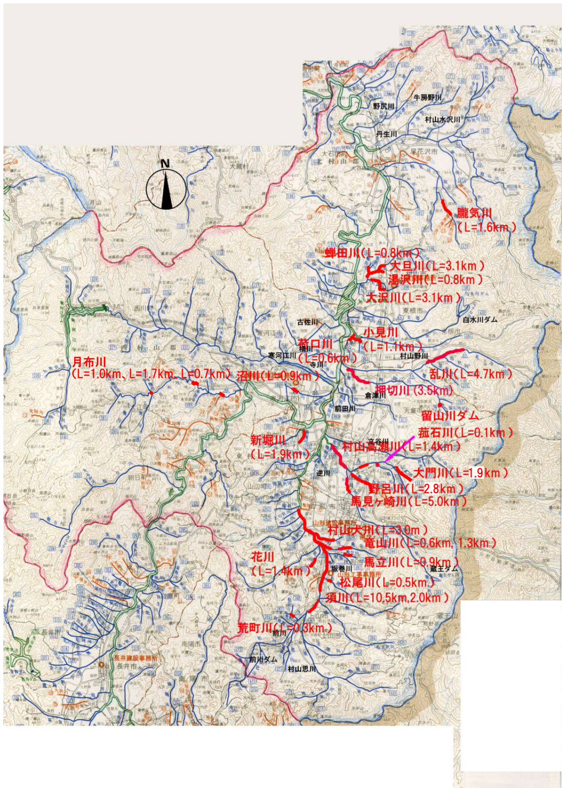
図1 施行河川位置図
