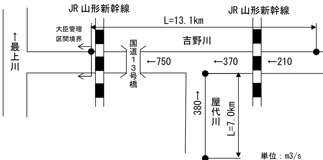
図8 計画流量配分図（吉野川、吉野川支川屋代川）
