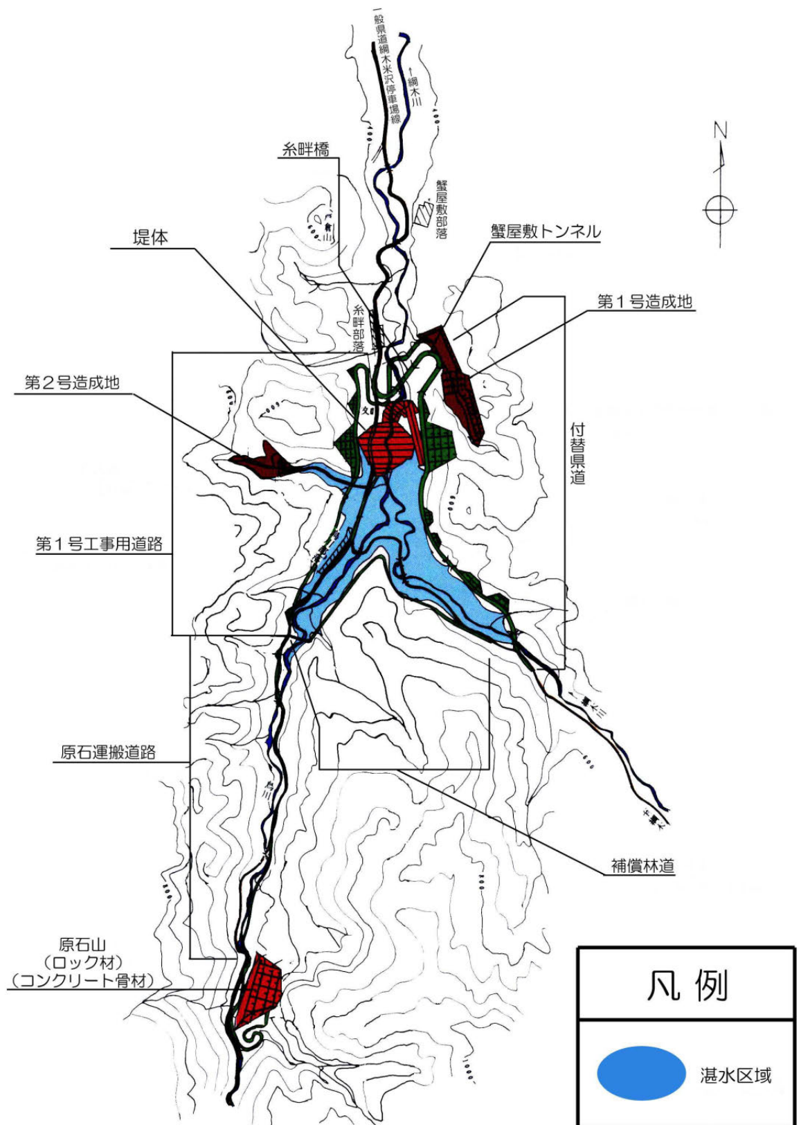
図 15 網木川ダム湛水区域図
