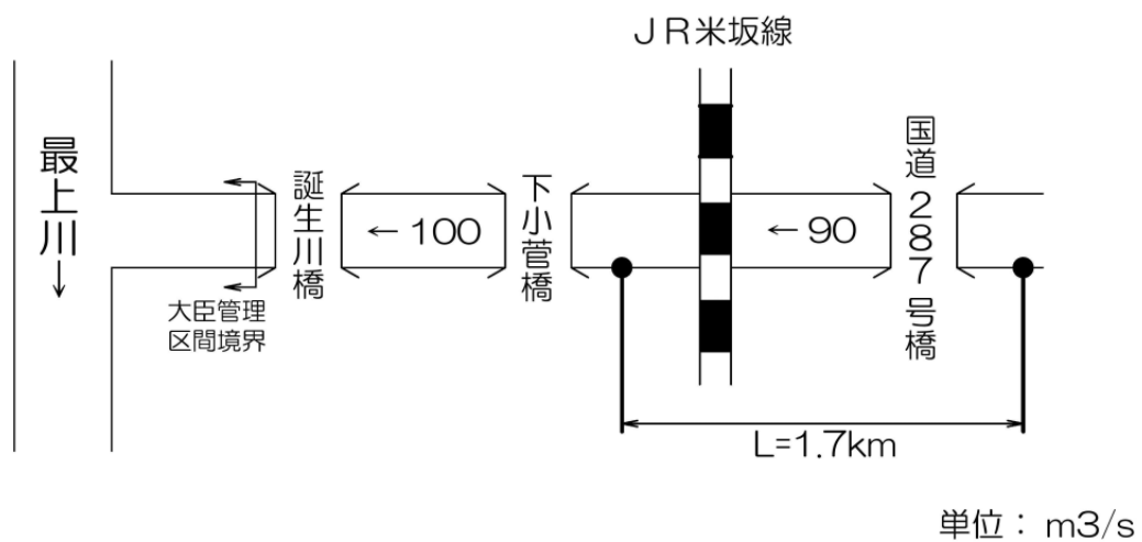
図6 計画流量配分図（誕生川）
