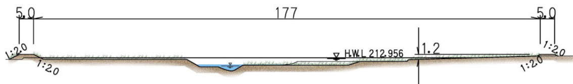
図 18 羽黒川代表断面図（最上川合流点から上流 0.5km、単位：m）
