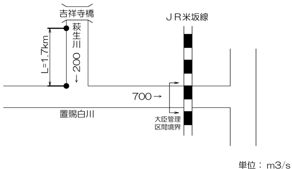
図4 計画流量配分図（置賜白川支川萩生川）
