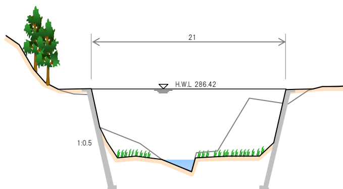
図 11 吉野川代表横断図（直轄管理区間から上流 12.3km、単位：m）
