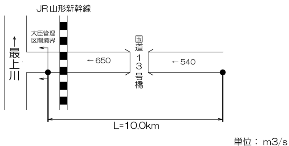
図 17 計画流量配分図（羽黒川）
