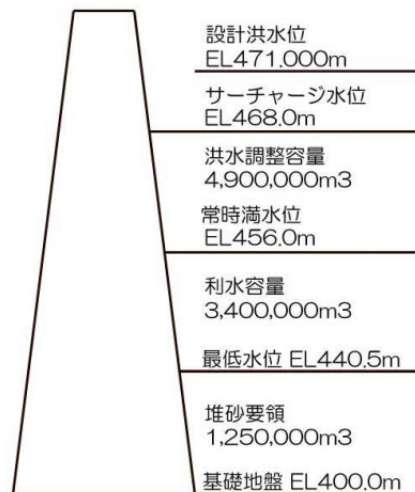
図 14 貯水池容量配分図
