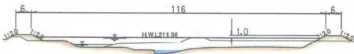
図 9 吉野川代表横断図（直轄管理区間から上流 0.1km、単位：m）
