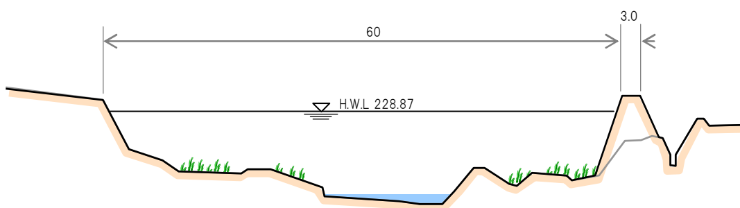
図 10 吉野川代表横断図（直轄管理区間から上流 5.0km、単位：m）
