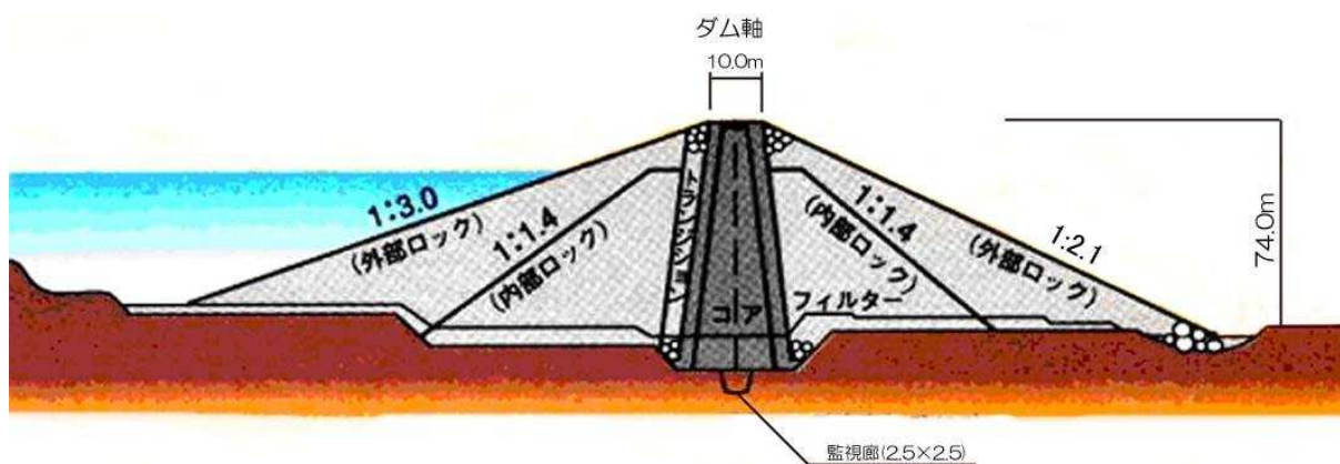
図 16 綱木川ダム堤体断面図
