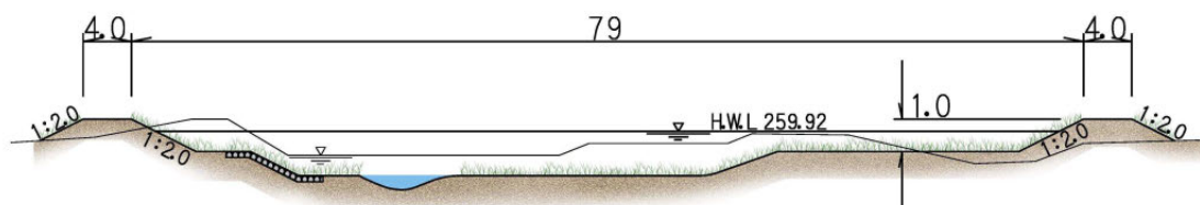
図 18 羽黒川代表断面図（最上川合流点から上流 0.5km、単位：m）
