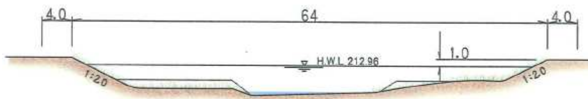
図 12 屋代川代表横断図（吉野川合流点から上流 0.3km、単位：m）
