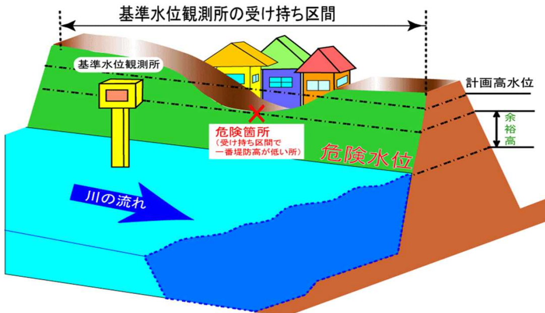
危機管理型水位計設置状況 (令和4年度末時点)
