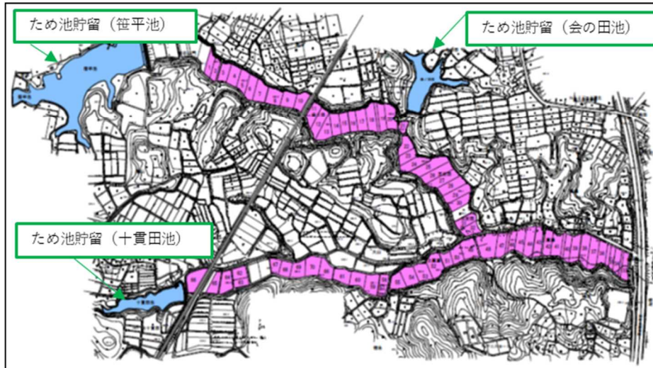
田んぼダム整備済平面図(令和2年度末)
