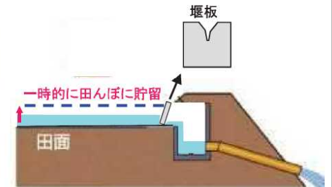
田んぼダム堰板の例
