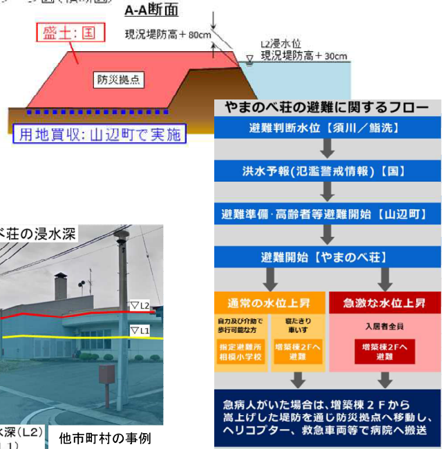
防災拠点イメージ図(横断面)
